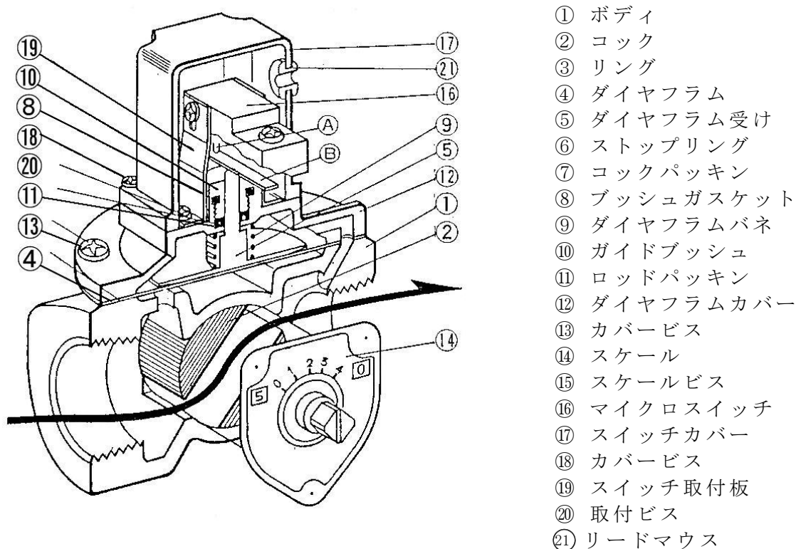
図1 フロースイッチ BN-1311-20A~40A
