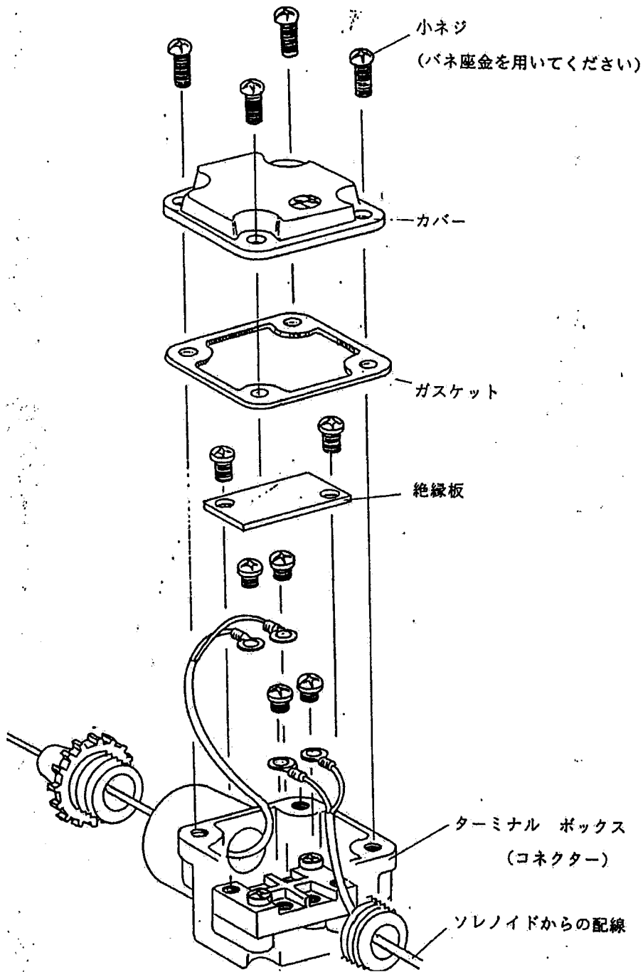
図2 防水型ターミナルボックス
